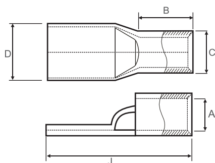
Cable Size 800 / 1000
